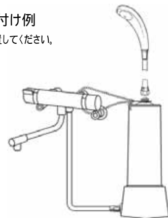
混合栓本体にボールチェーンを取り付ける方法
